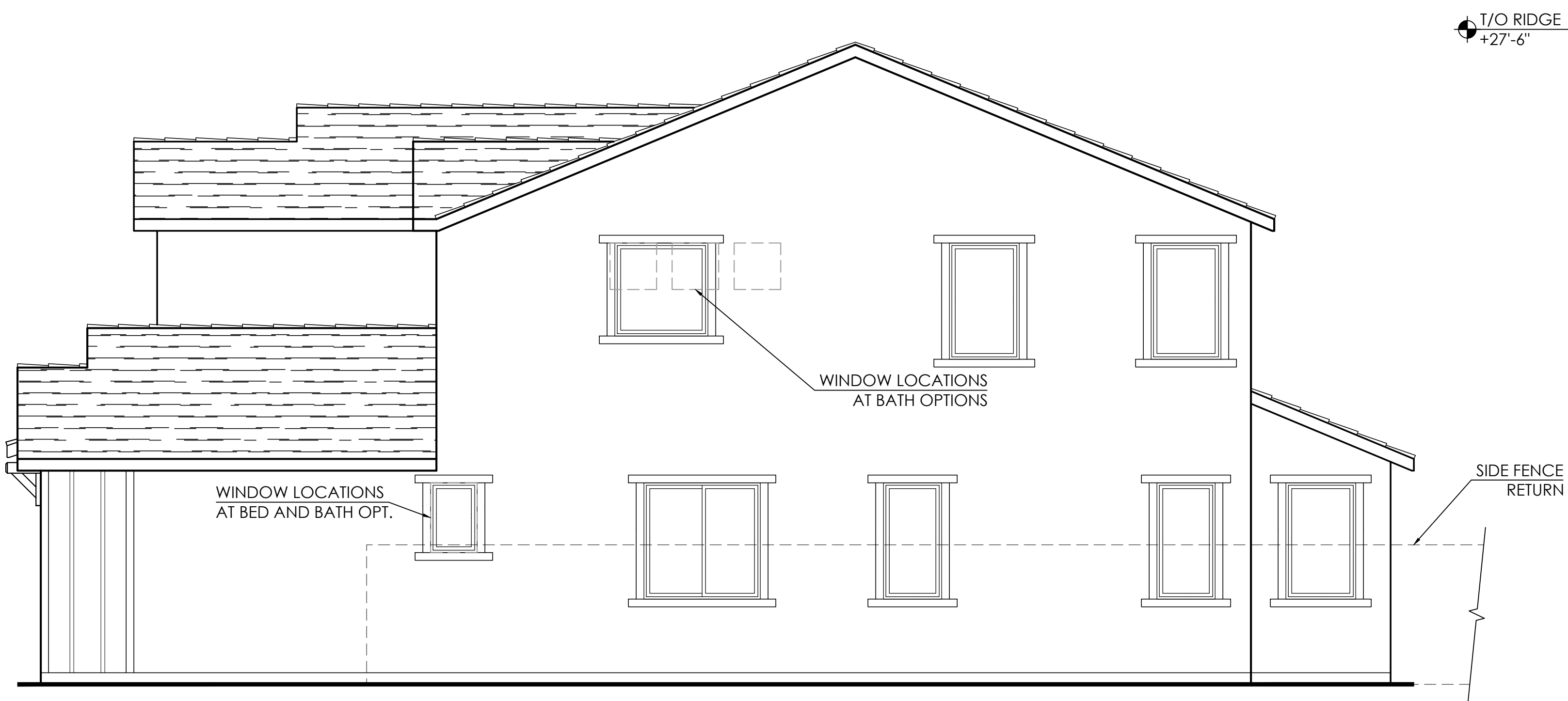
Right Elevation
