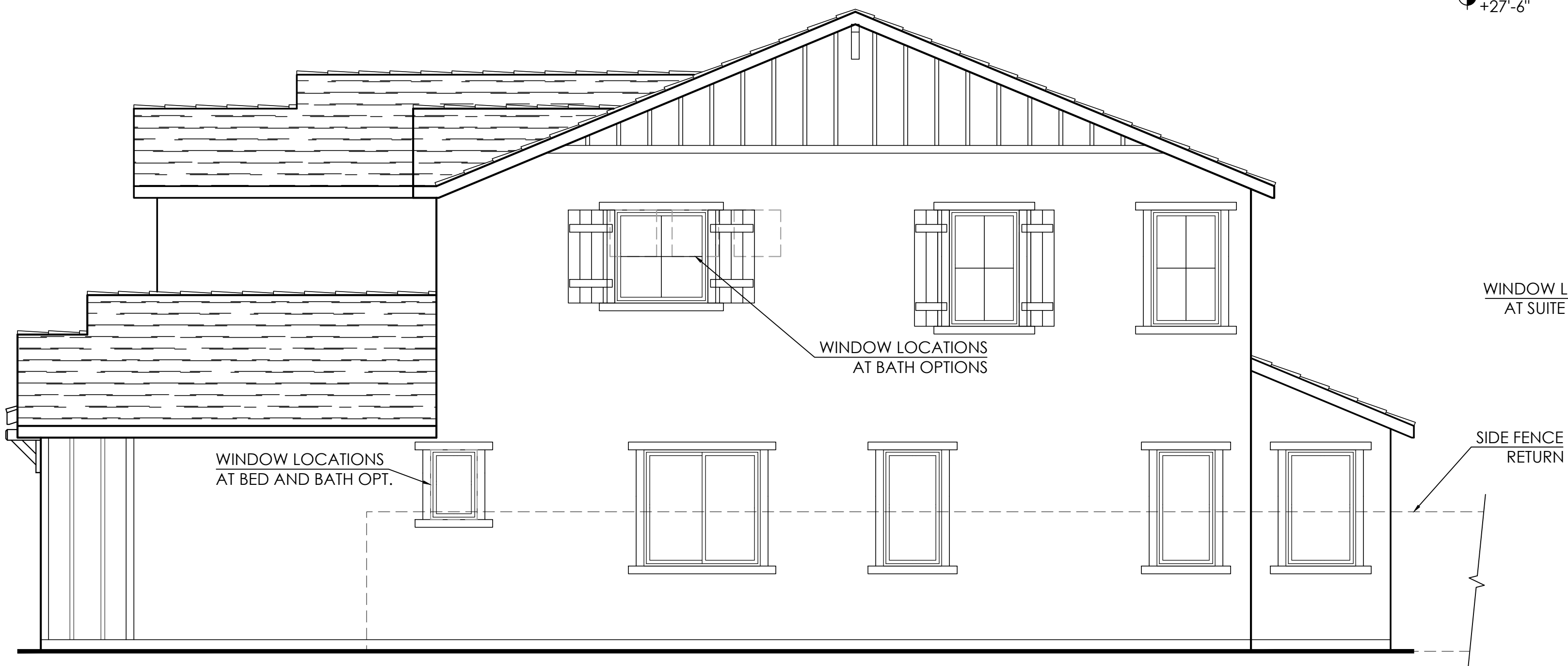
Right Elevation
