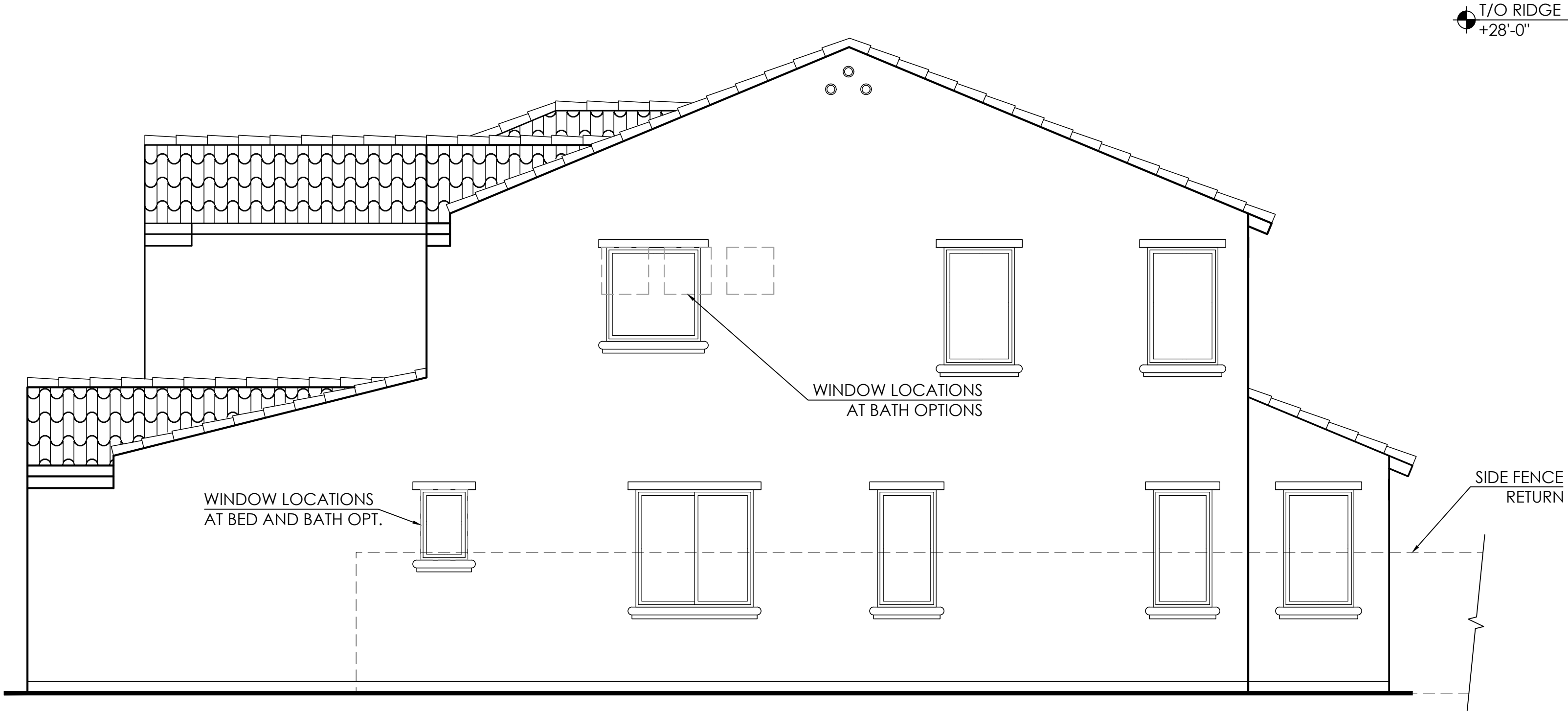
Right Elevation
