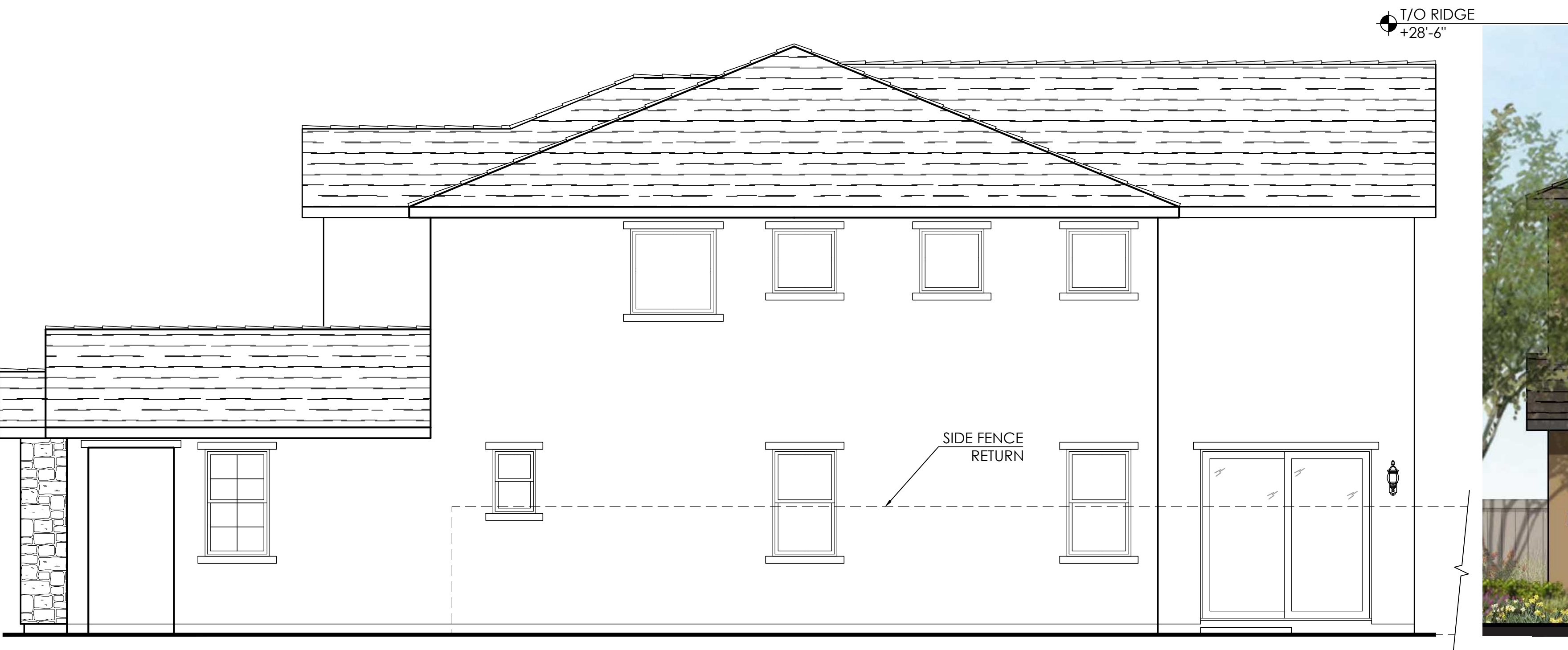
Right Elevation
