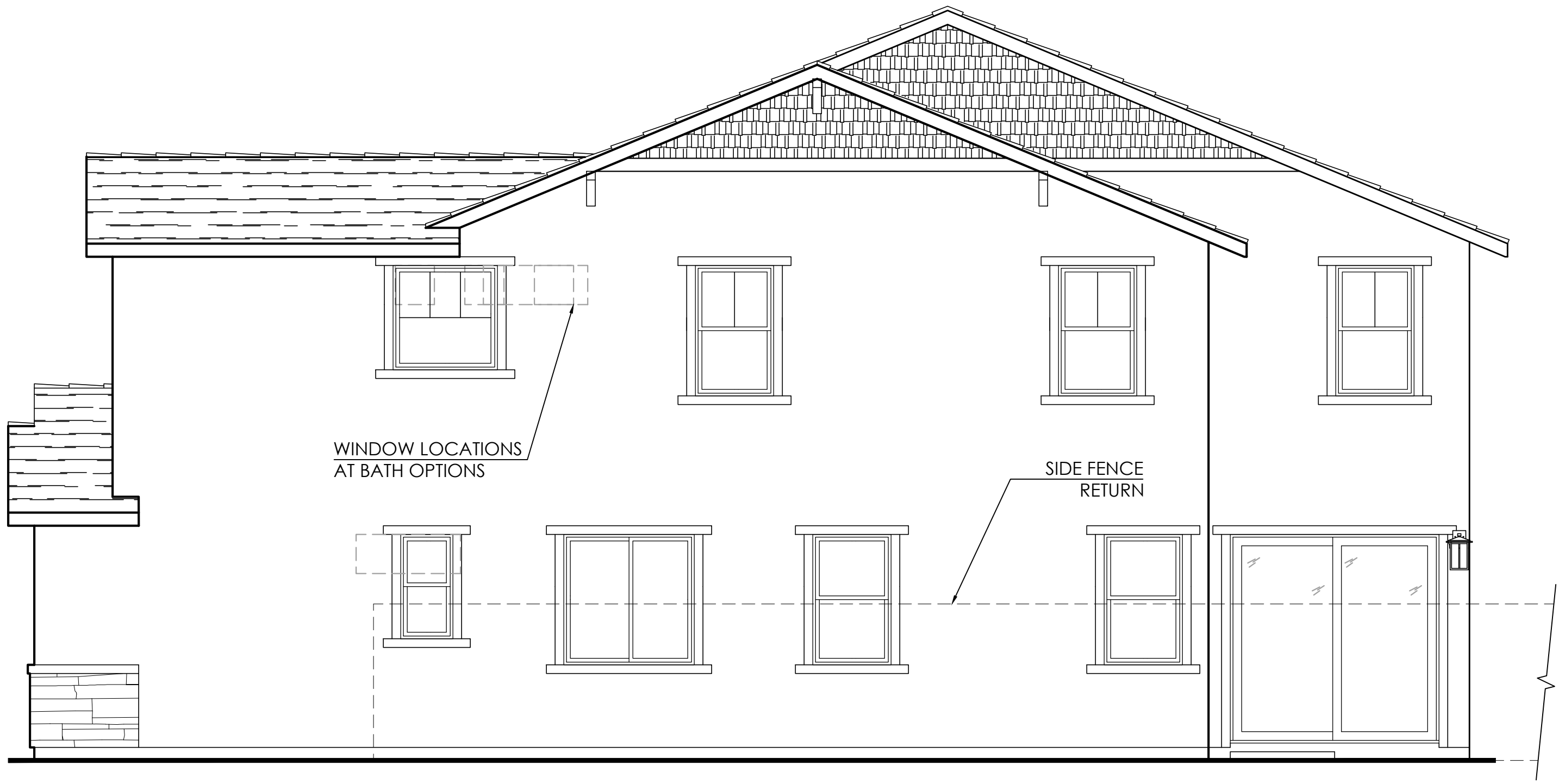
Right Elevation
