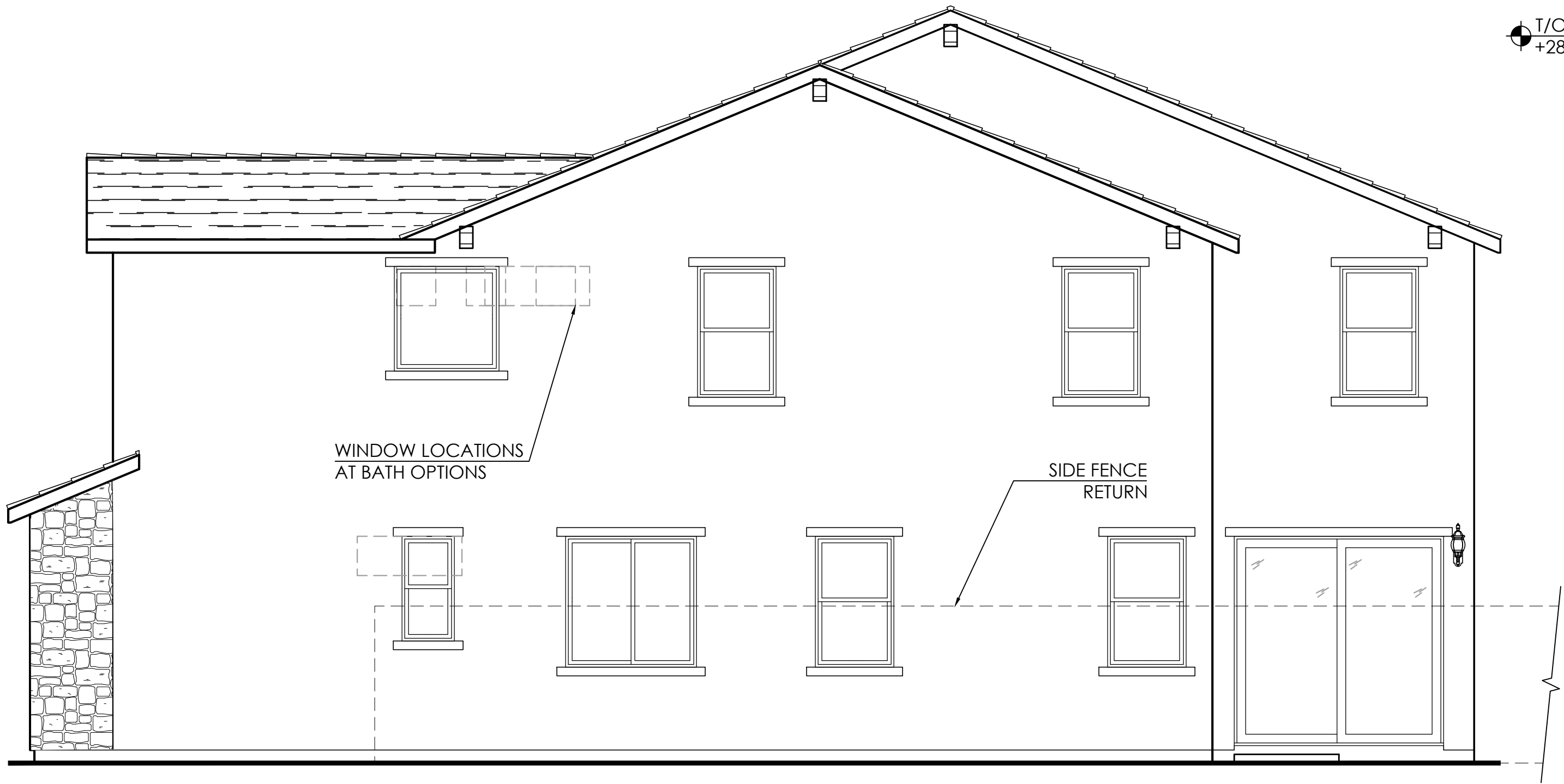
Right Elevation
