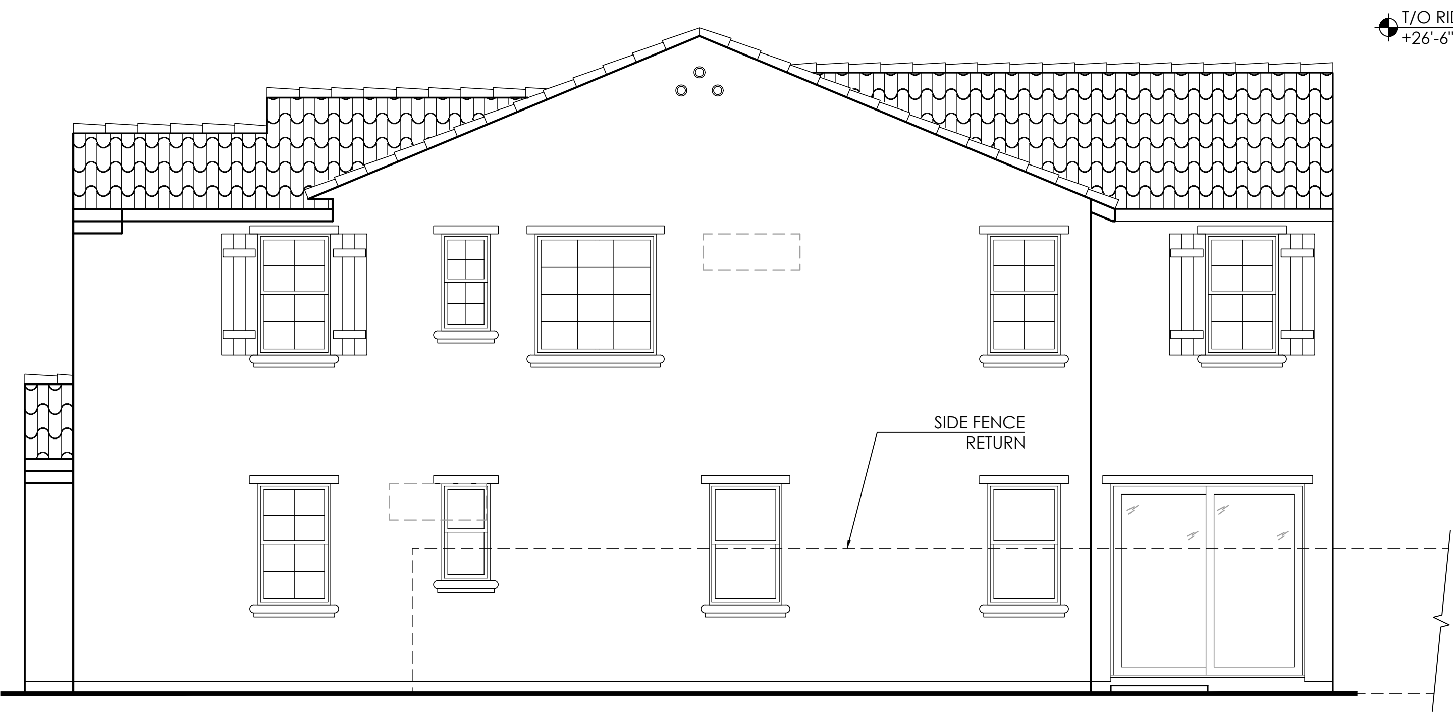
Right Elevation
