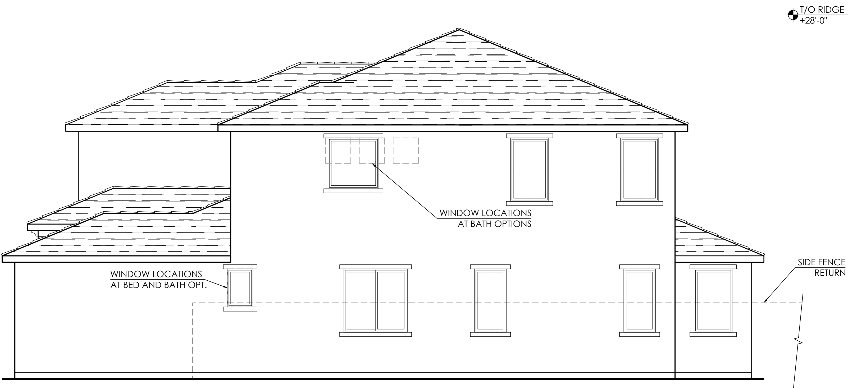
Right Elevation
