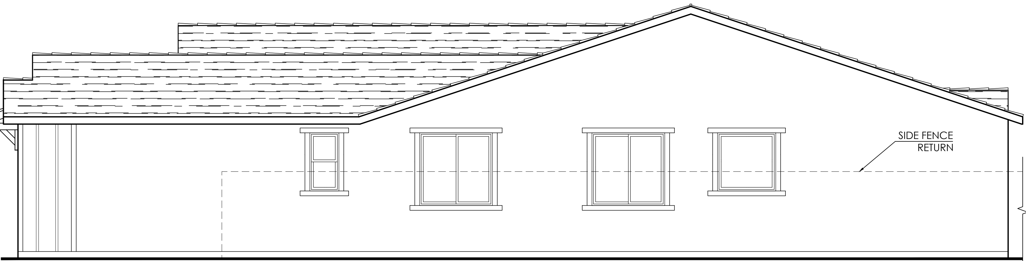
Right Elevation
