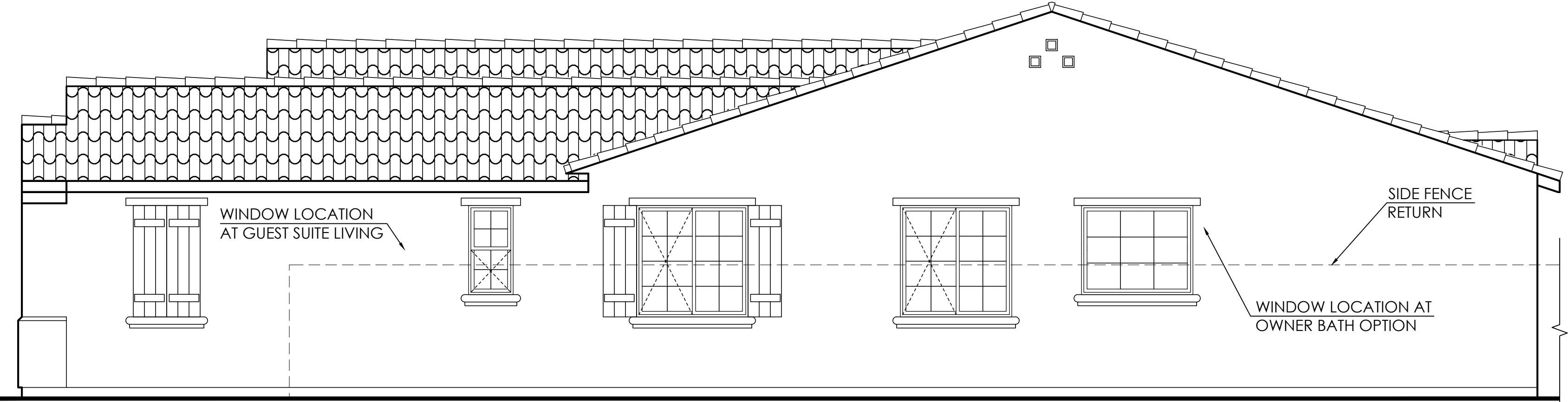
Right Elevation
