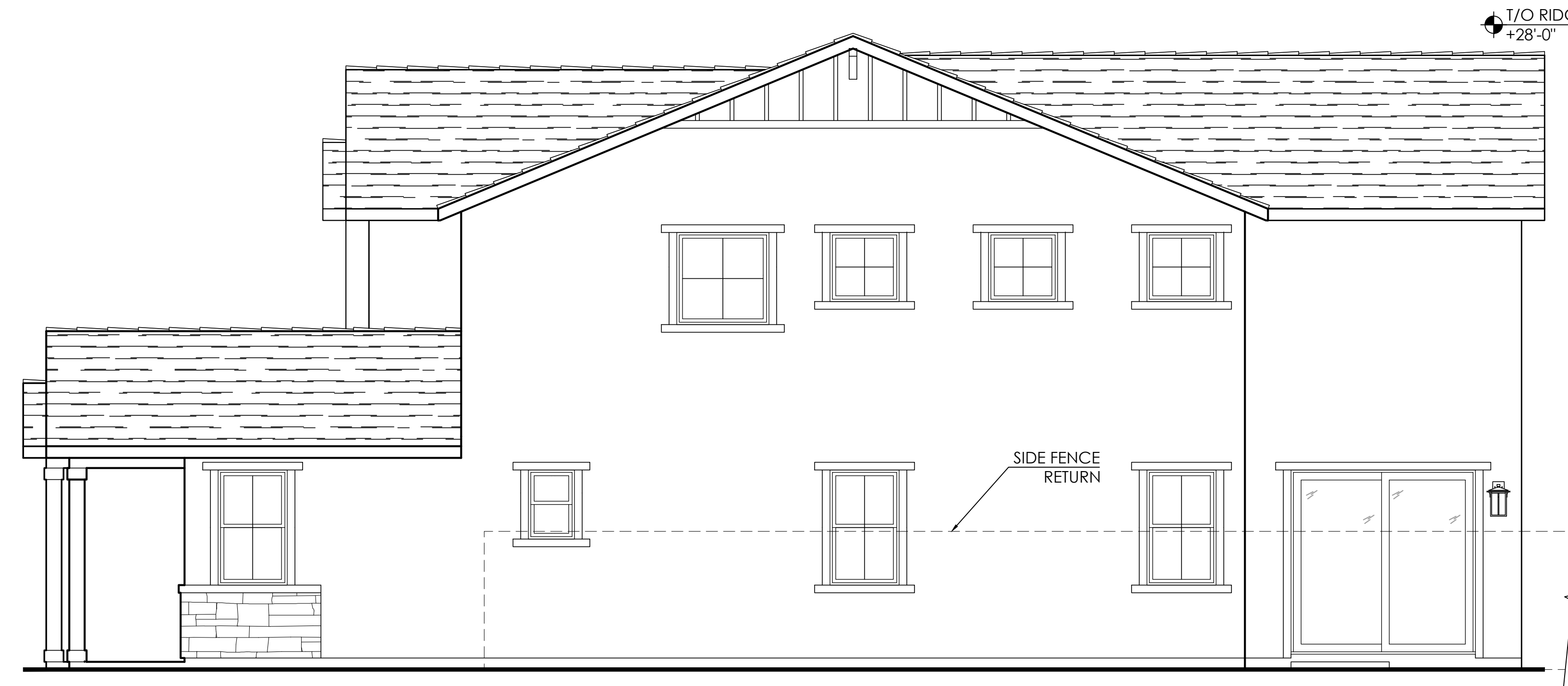
Right Elevation
