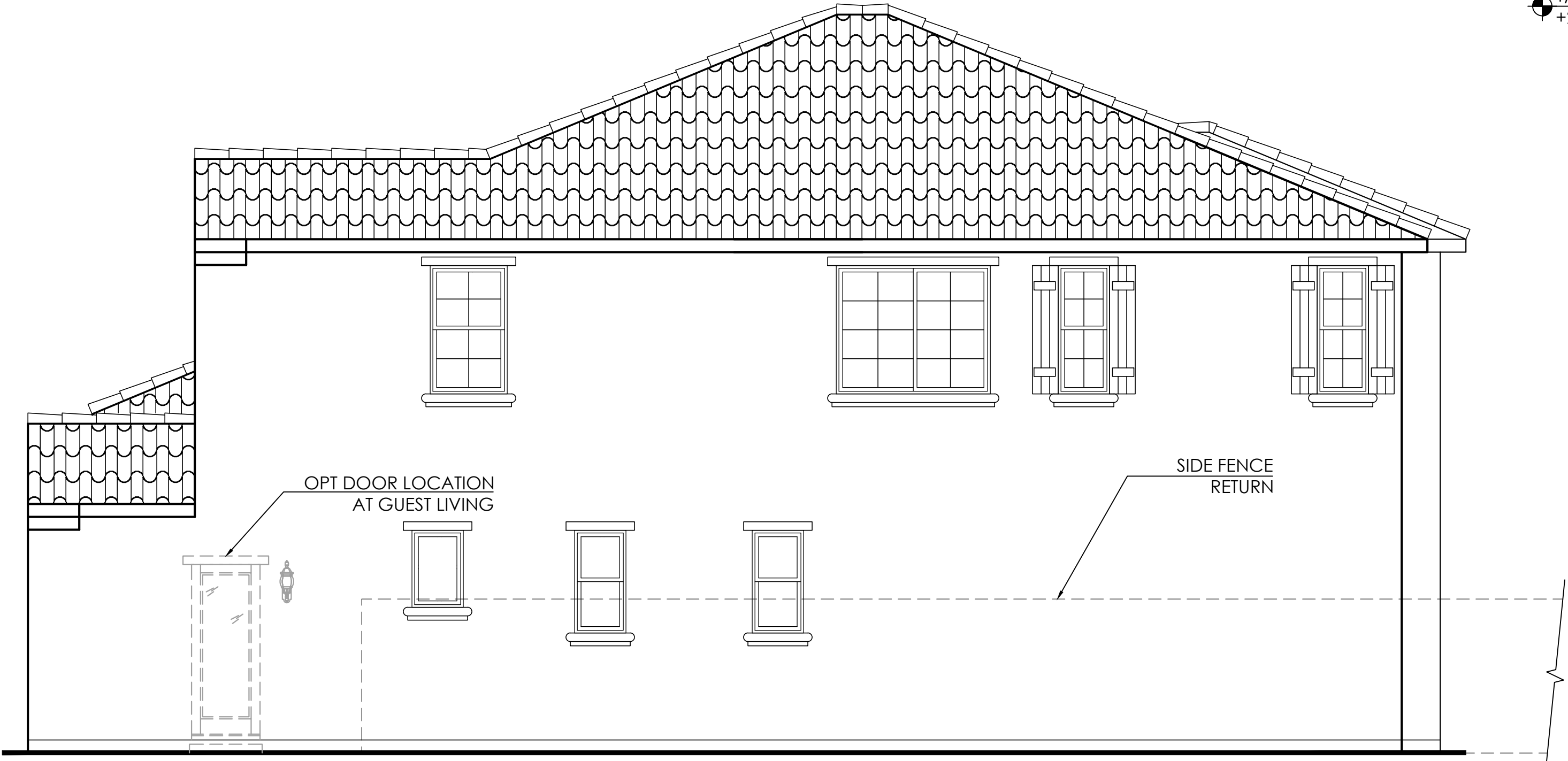
Right Elevation
