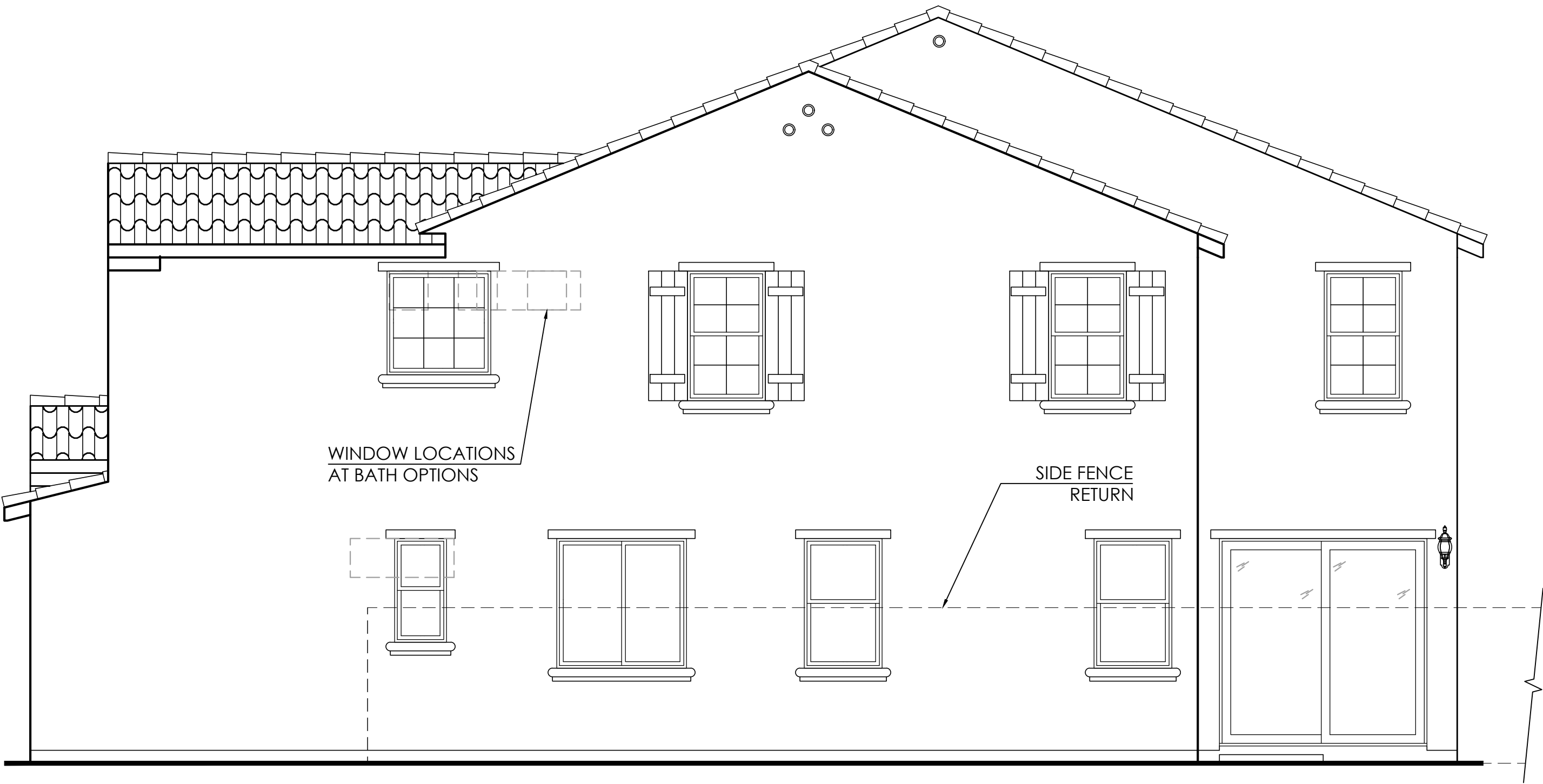
Right Elevation
