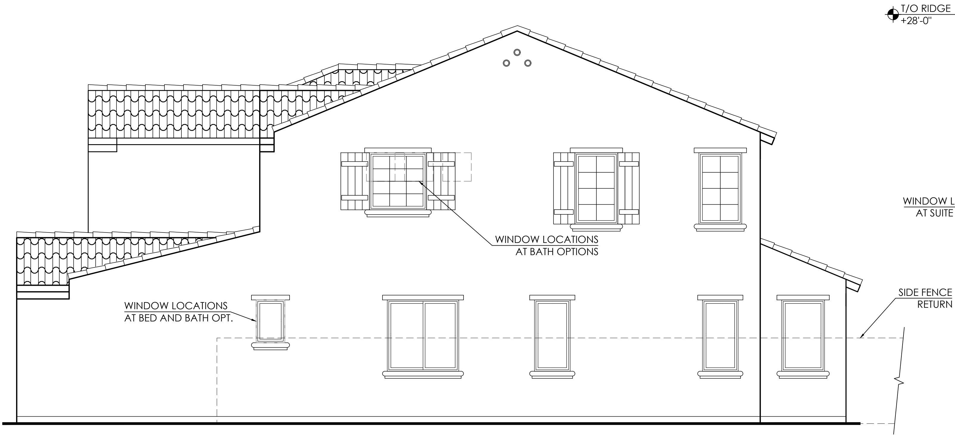
Right Elevation
