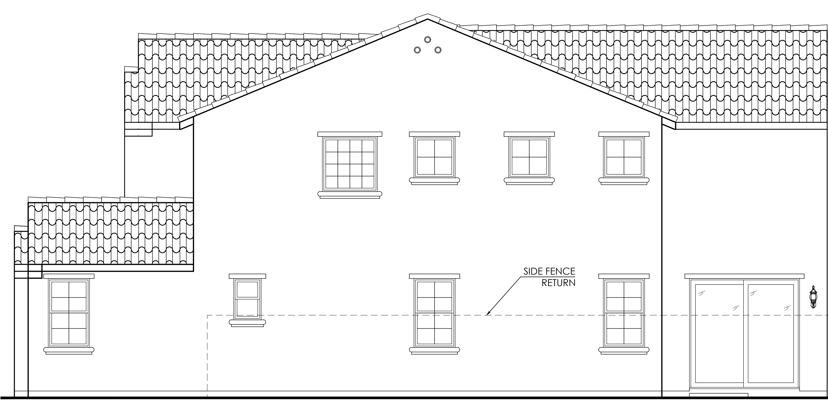
Right Elevation
