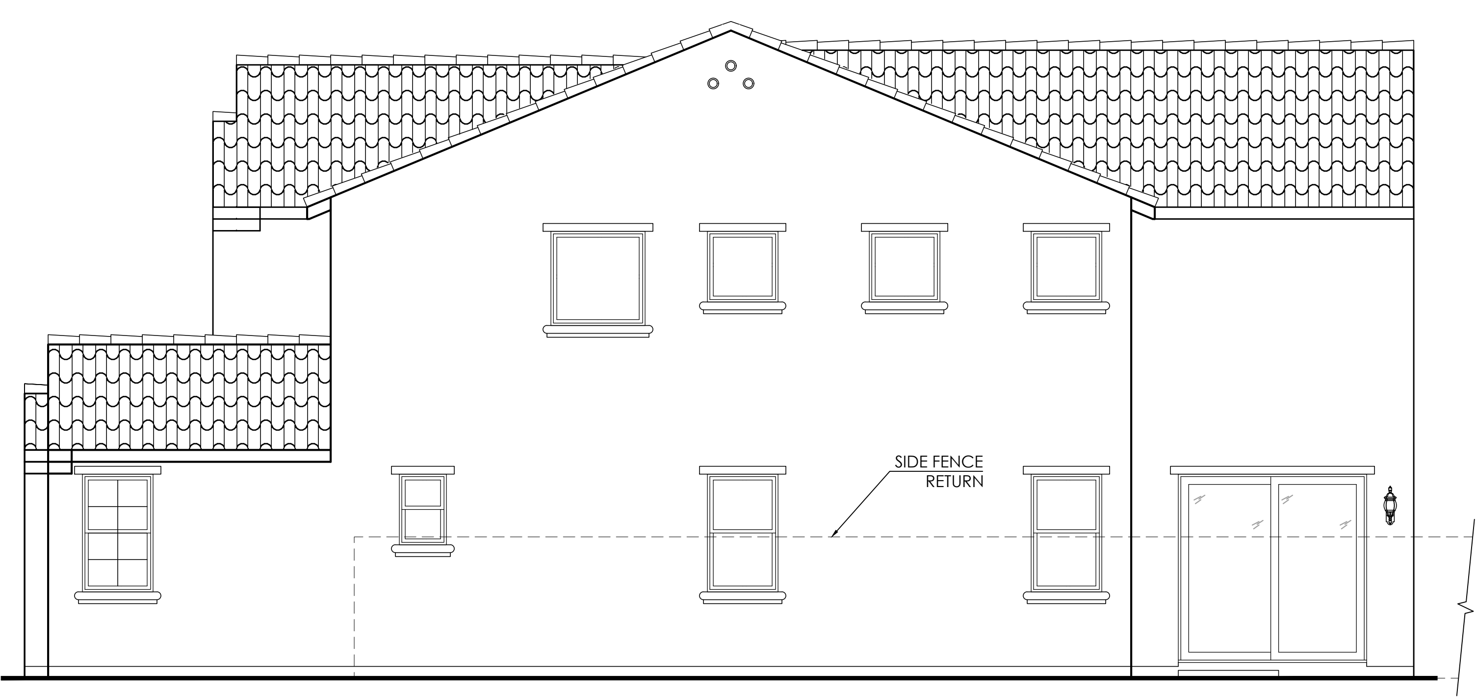
Right Elevation
