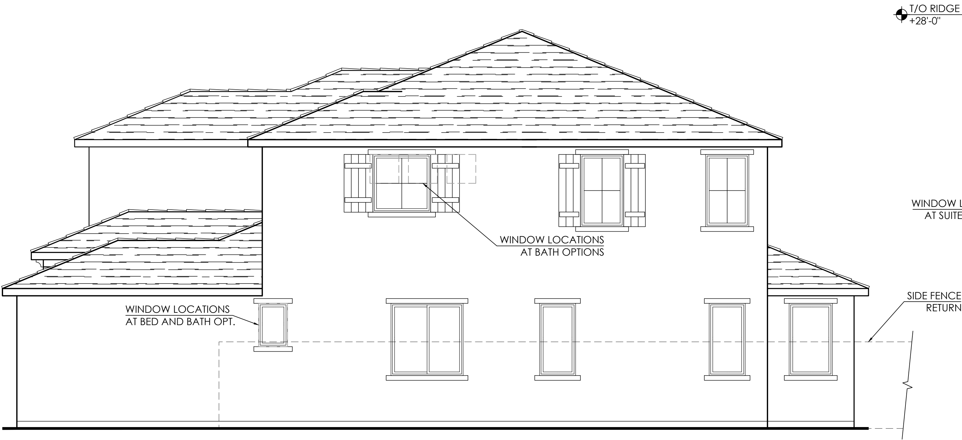
Right Elevation
