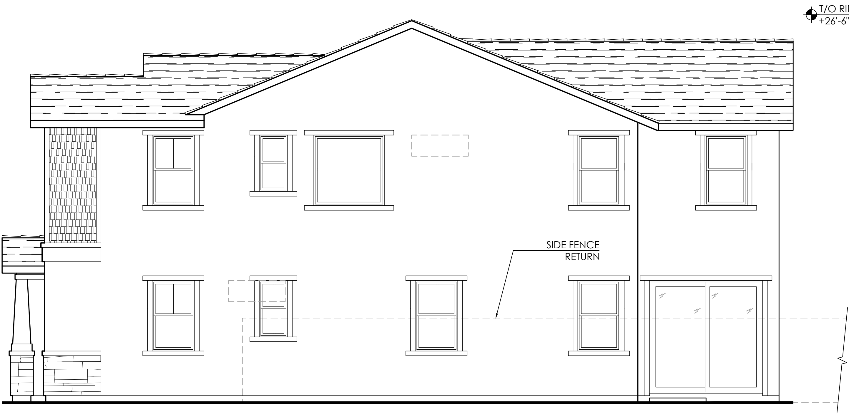
Right Elevation
